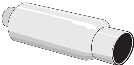
U 28 63 02R Slutdämpare "SPRINT 63 XL" Rund/round 140 mm, L=400 mm (excl. muffar/ends) Ändrör/tailpipe: 114 mm, rullad kant Med upphängningsband/With hanging strap
