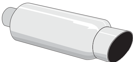
U 28 63 03R Slutdämpare "SPRINT 63 JAP" Rund/round 140 mm, L=400 mm (excl. muffar/ends) Ändrör/tailpipe: 114 mm, snedsågat/skewed Med upphängningsband/With hanging strap
