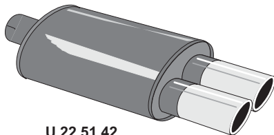
U 22 51 42 Slutdämpare/Rear silencer "MAXI" Oval 100/165 mm, L=250 (excl. muffar/ends) Totallängd/total length = 540 mm (incl. ändrör/tailpipes) Ändrör/tailpipes: 2x58 mm Med upphängningsögla/With hanging point
