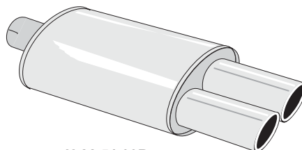
U 22 51 00R Slutdämpare/Rear silencer "MAXI" Oval 100/165 mm, L=250 (excl. muffar/ends) Totallängd/total length = 540 mm (incl. ändrör/tailpipes) Ändrör/tailpipes: 2x58 mm Med upphängningsögla/With hanging point
