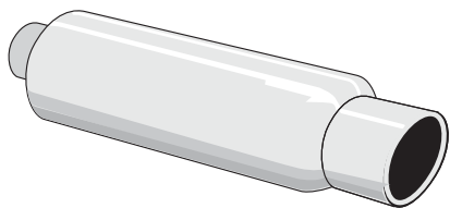
U 28 63 01R Slutdämpare "SPRINT 63" Rund/round 125 mm, L=400 mm (excl. muffar/ends) Ändrör/tailpipe: 100 mm, rullad kant Med upphängningsband/With hanging strap
